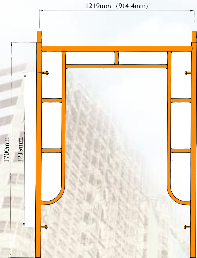
BEATTY FRAME
